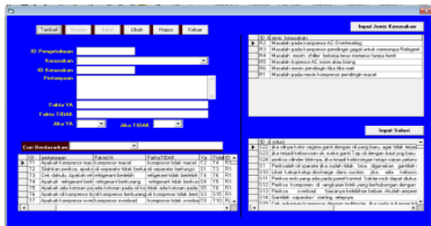
Gambar 11. Form pengetahuan
